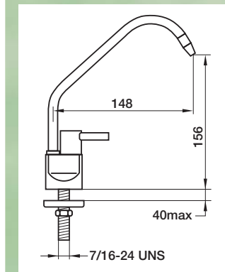
Art. DERBY - IN ACCIAIO INOX - 1 VIA
